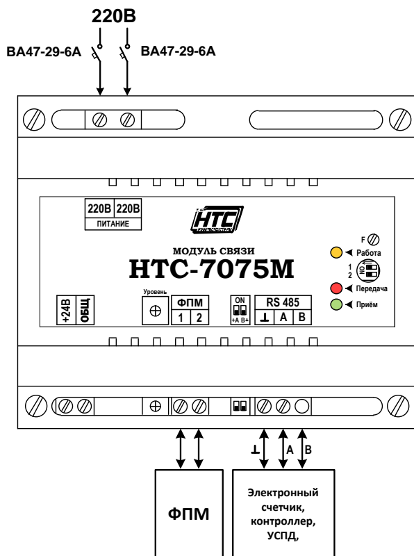
Рис.1. Схема подключения модуля связи НТС-7075М. 35
