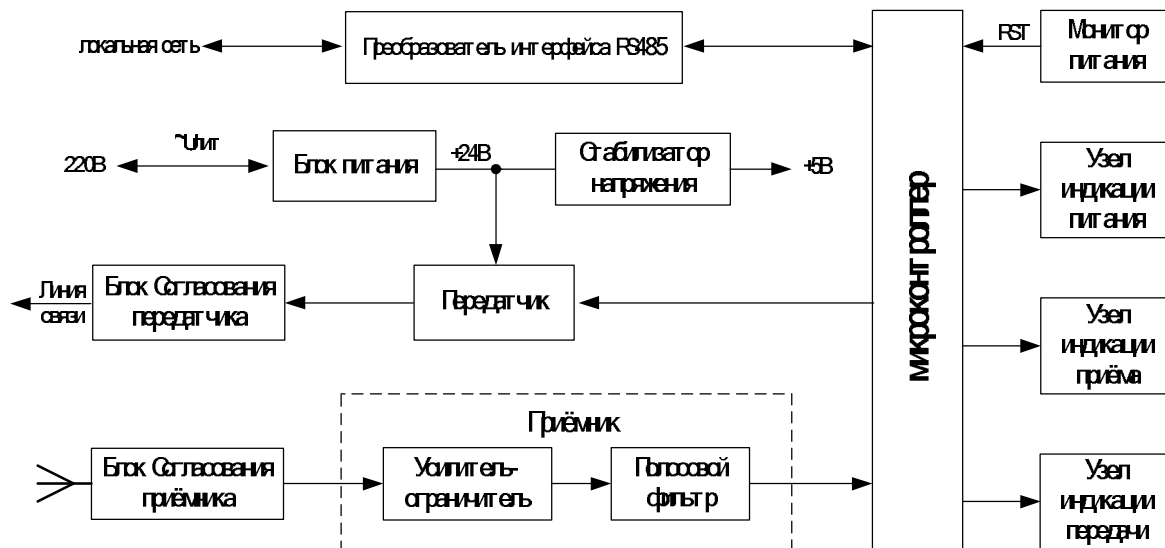
Рисунок 2. Структурная схема модуля связи НТС-7075.02
