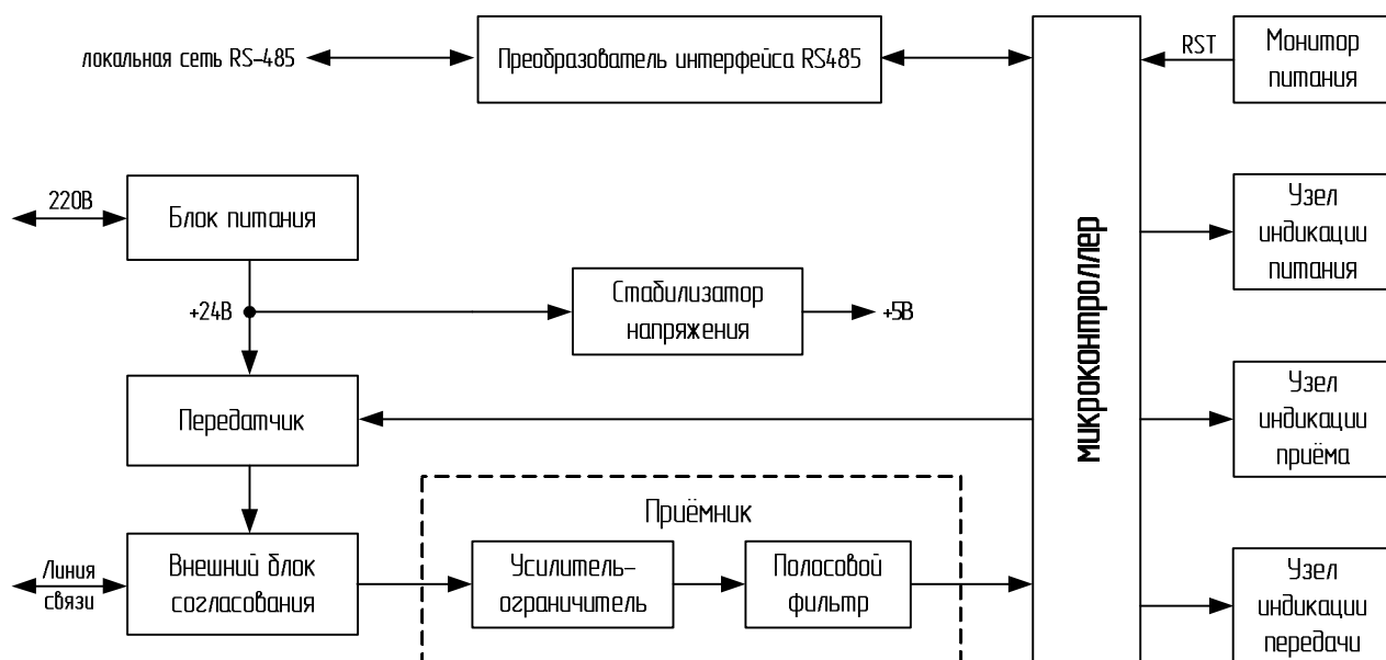
Рисунок 2. Структурная схема модуля связи НТС-7075-05
