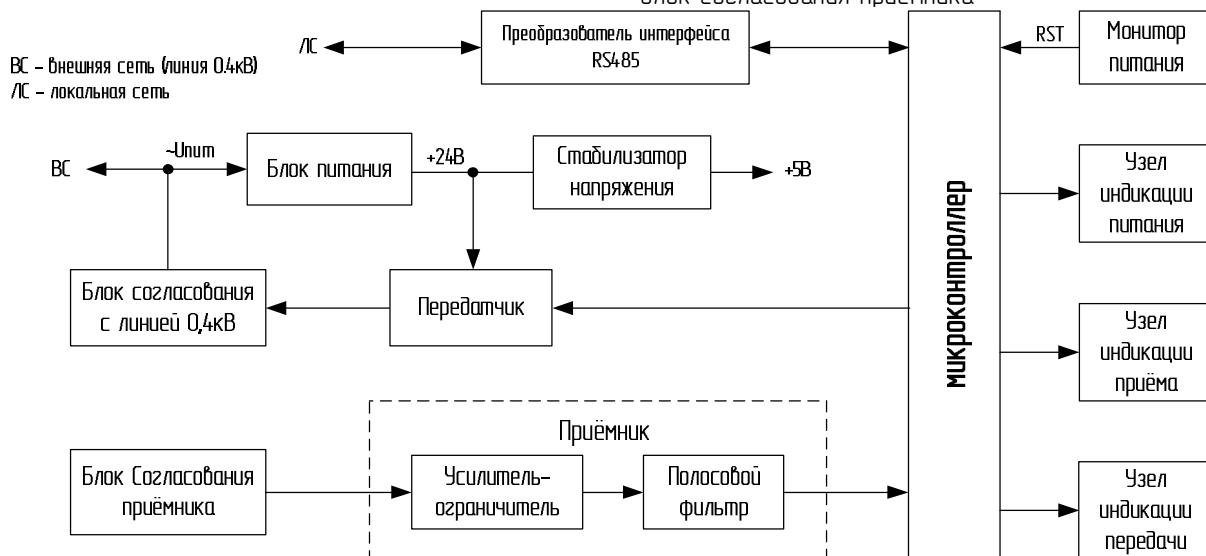
Рисунок 2. Структурная схема модуля связи НТС-7075-03
