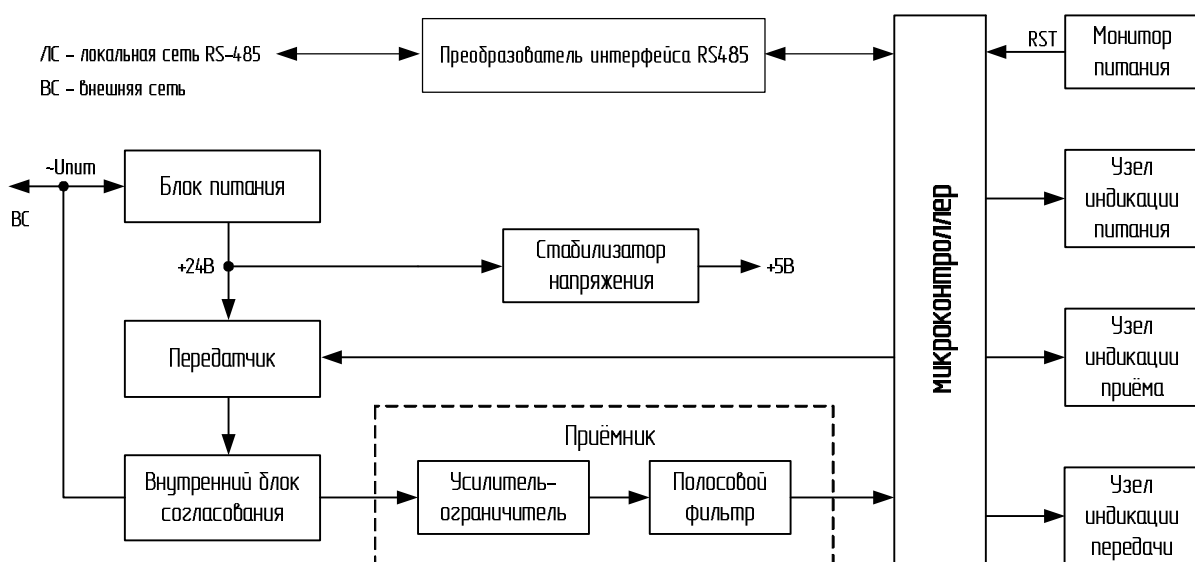
Рисунок 2. Структурная схема модуля связи НТС-7075-01
