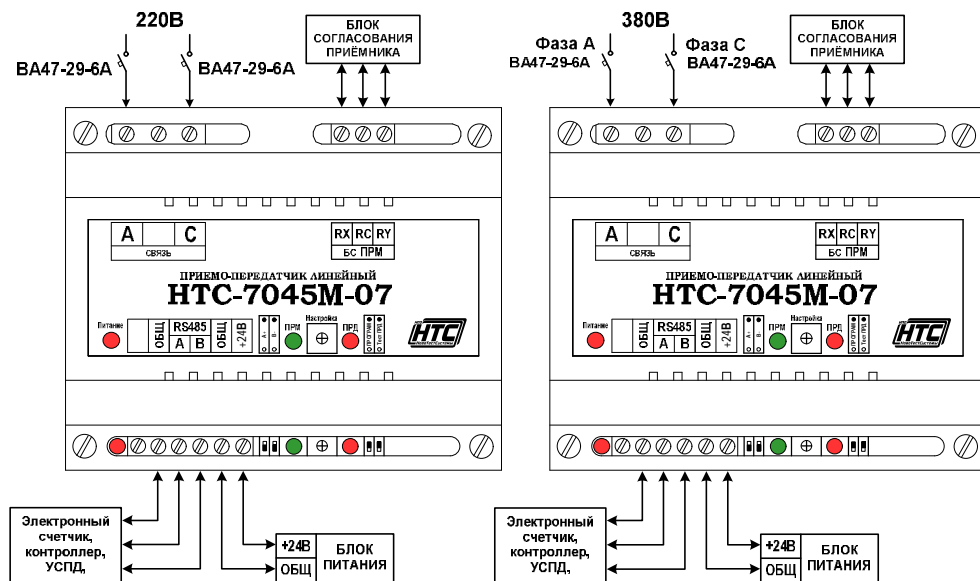
Рис.1. Схемы подключения приёмно-передатчика линейного HTC-7045M-07.
